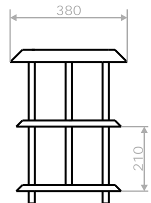
Vista lateral
